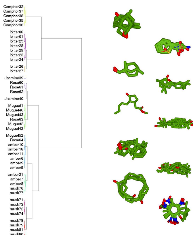
Figure 4.25: Le clustering de forme de surface SH de l'ensemble de données d' Odour . À gauche : le dendrogramme obtenu en utilisant des calculs de similarité de forme SH avec L=6 . À droite : les superpositions correspondantes 3D moléculaires.
