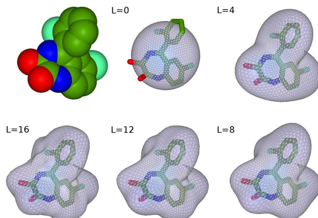
Figure 2.10: Les surfaces SH de lorazépam à divers ordres d'expansion.
