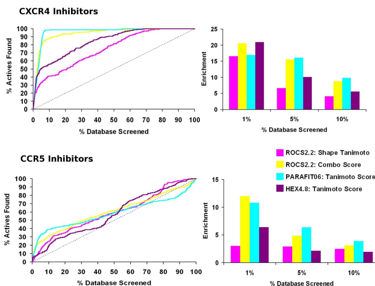
Figure 4.27: Des courbes d'enrichissement de VS pour les inhibiteurs de CXCR4 et CCR5. Les courbes d'enrichissement sur la gauche montrent une capacité relative des programmes ROCS, ParaFit et Hex d'identifier des inhibiteurs connus à partir d'une base de données de molécules inhibitrices et de leurre pour les protéines CXCR4 et CCR5. La ligne pointillée représente l'enrichissement qui aurait été obtenu si des inhibiteurs étaient retrouvés au hasard. Les diagrammes à barres sur la droite montre des EF pour les premiers, 1%, 5% et 10% des bases de données criblées.
