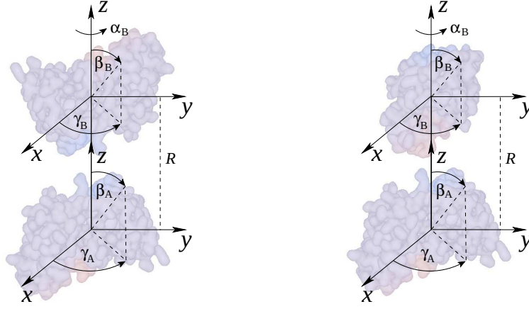
Figure 4.1: Une illustration schématique des espaces de recherche en corps rigide 6D d'appariement de forme (à gauche) et d'amarrage (à droite) en termes d'une coordonnée de translation, R , et de cinq coordonnées de rotation d'Euler, (\beta_A, \gamma_A) et (\alpha_B, \beta_B, \gamma_B) , assignées au récepteur et au ligand, respectivement. La distance entre les centres moléculaires sera petite et deux des angles de rotation seront presque redondants.
