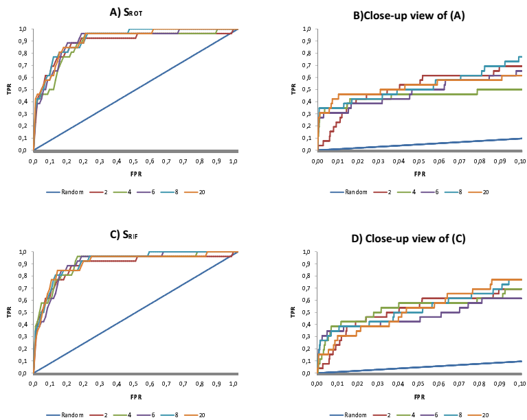
Figure 4.8: Les analyses des courbes ROC obtenues en interrogeant la base entière de données CATH avec la structure 12asA00. A : (ROT) fonction de score rotation-dépendante, Eq 4.11; B : vue en gros plan de (A); C : fonction de score RIF, Eq 4.14; D : vue en gros plan de (C).
