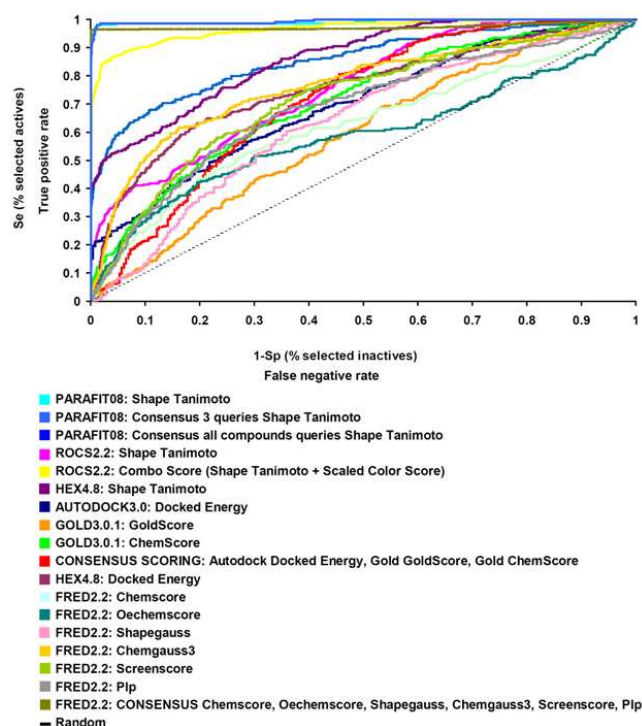
Figure 4.29: Les analyses des courbes de ROC de VS basé sur le ligand et le récepteur en utilisant AMD3100 et des requêtes de forme consensuelles des pseudo-molécules contre la base de données des inhibiteurs de CXCR4.
